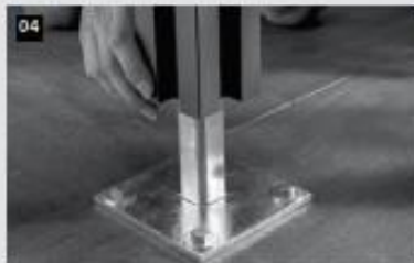
04 Pfosten-Anker zum Anschrauben Mit stabiler Schraubplatte, Pfosten wird auf Anker gesteckt / montiert
