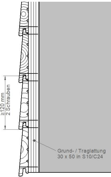
Keilprofil 26/14 mm
