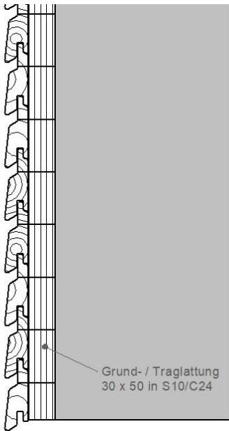
Befestigung Rhombusprofil 27 mm N+F
